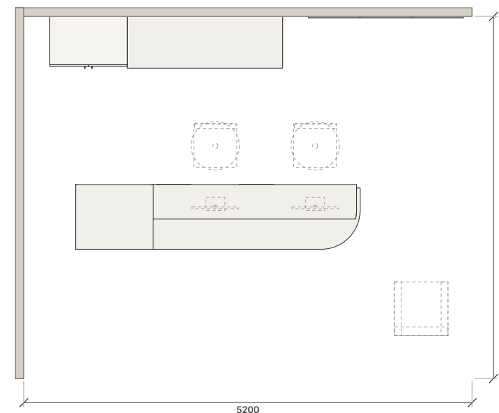
PLAN CAMERĂ · 1:62
