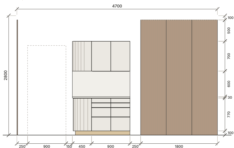
FAȚADĂ · 1:55
