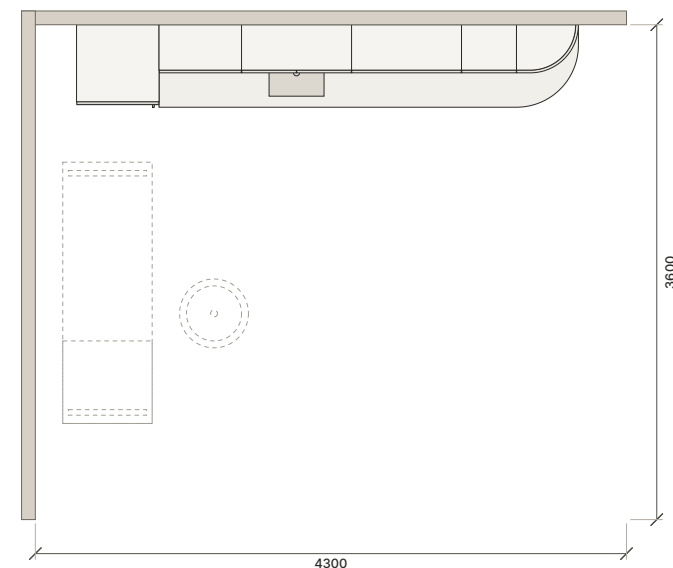
PLAN CAMERĂ · 1:55
