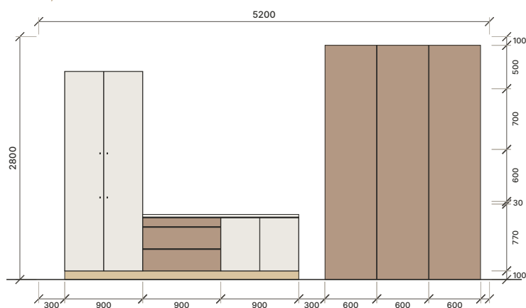
FAȚADĂ · 1:62
