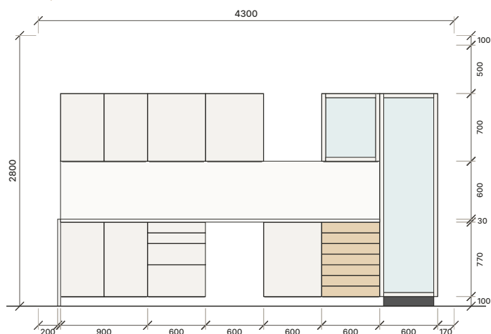
FAȚADĂ · 1:55
