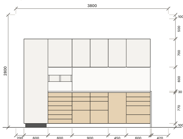
FAȚADĂ · 1:55
