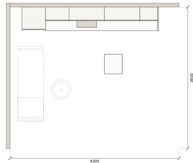
PLAN CAMERĂ · 1:55
