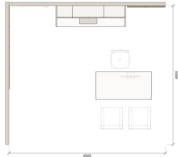
PLAN CAMERĂ · 1:55
