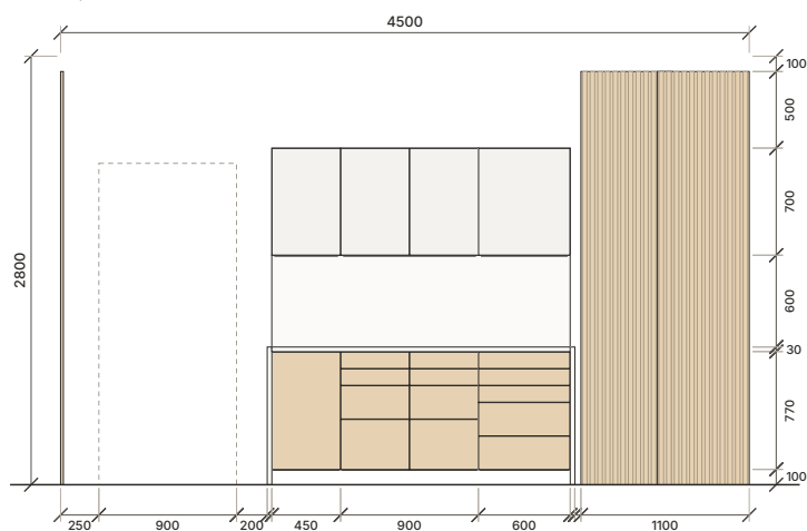
FAȚADĂ · 1:55
